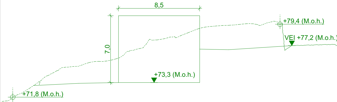
Snitt Y
