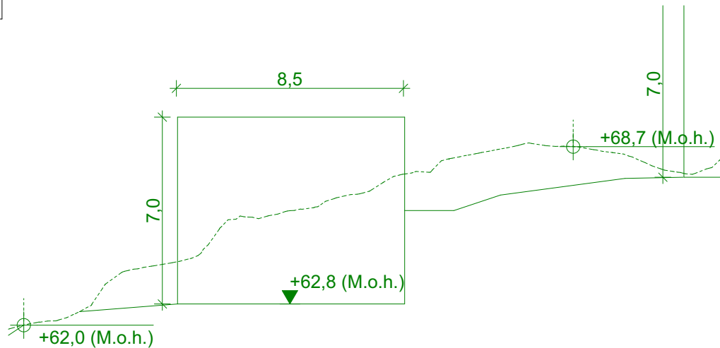
Snitt Y
