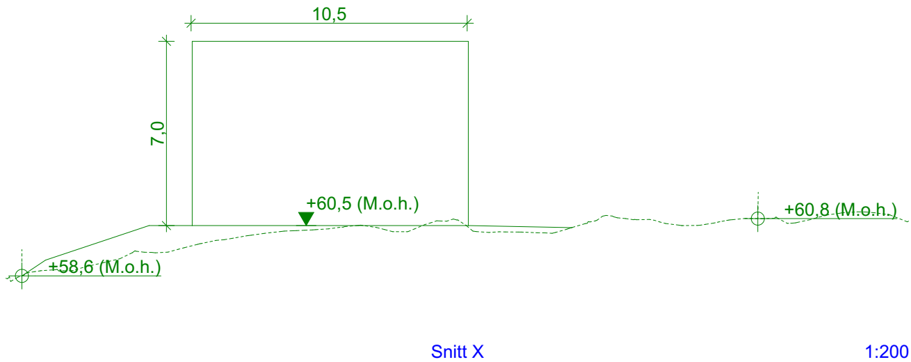
SNITT X-X
