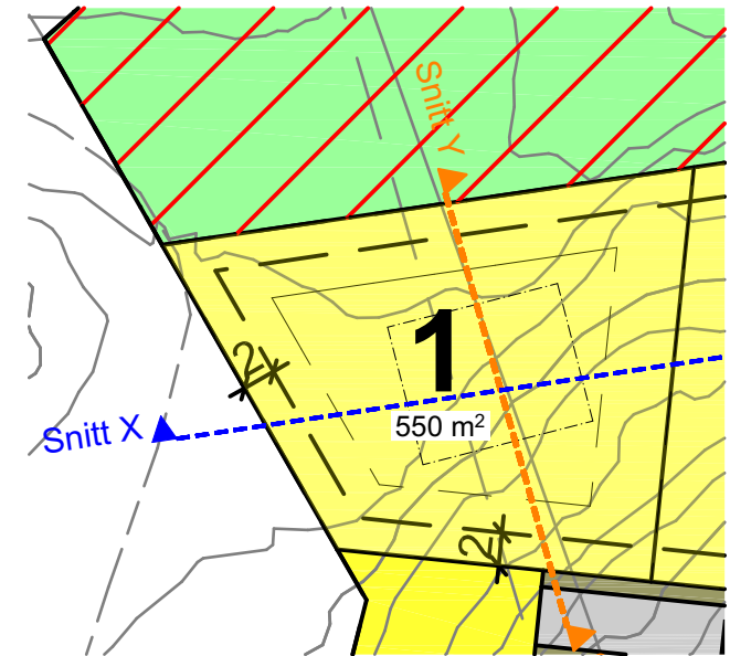
UTDRAG TOMTEPLAN 1:500
