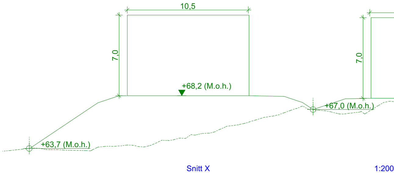
SNITT X-X
